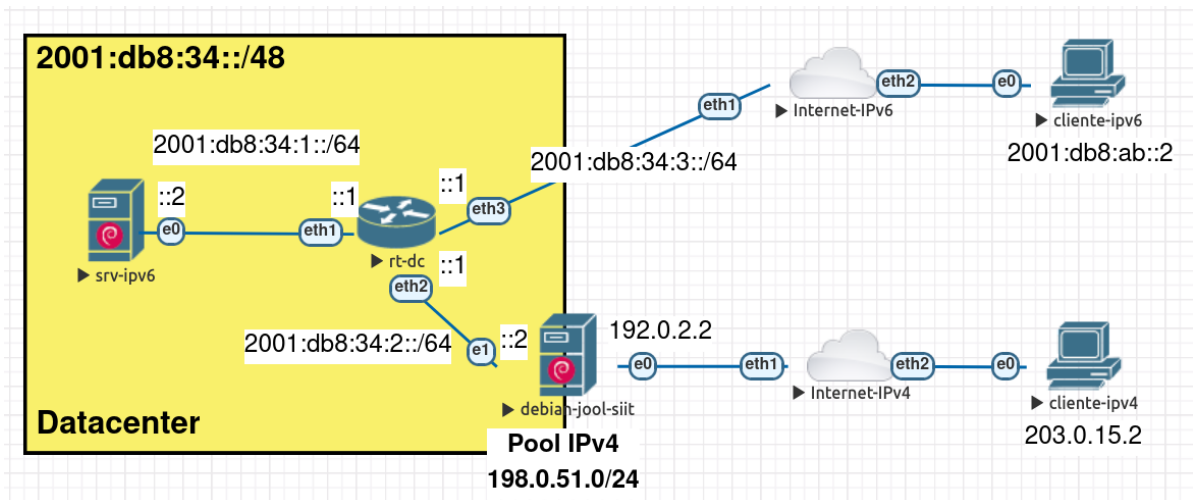
Fig. 1: Topologia SIIT-DC
