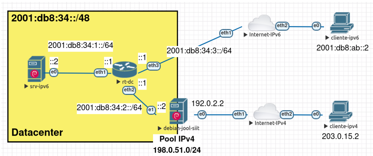
Fig. 1: Topologia SIIT-DC
